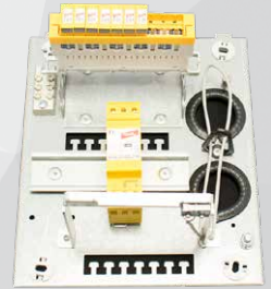
Montageplatte bestückt (inkl. Ausbaureserve, z. B. für FAT/FBF)
